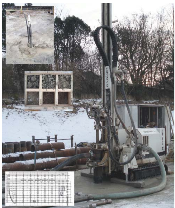
▼ Bohrgerät und Darstellung des Lageplanes des Erdwärmesondenfeldes, Fächerkiste mit Bohrproben und einer eingebauten Erdwärmesonde
